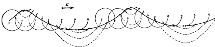
Рис. 437. Связь линий тока и круговых путей в бегущих водяных волнах. Горизонтальный ряд точек показывает частицы поверхности воды в состоянии покоя, дуги окружностей — пути, пробегаемые ими по направлению часовой стрелки. Соединив маленькие острия стрелок , мы получаем профиль распространяющейся вправо волны в конце следующего промежутка времени. Круговые траектории вычерчены для каждой второй стрелки.
