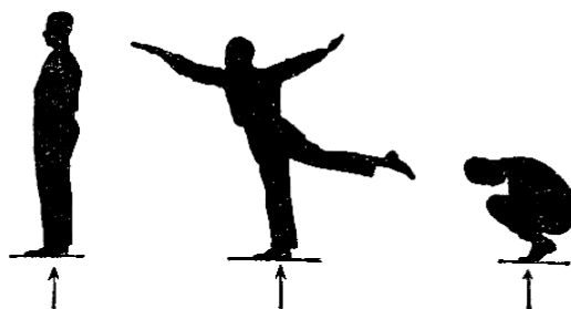
Рис. 124. \Theta = 1,2 \text{ кг} \cdot \text{м}^2 . Рис. 125. \Theta = 8 \text{ кг} \cdot \text{м}^2 . Рис. 126. \Theta = 2,3 \text{ кг} \cdot \text{м}^2 . Рис. 124—126. Моменты инерции человека в разных положениях. Стрелки показывают направление осей вращения.
