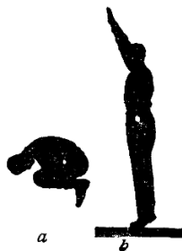
Рис. 138. Изменение момента инерции при сальто.
