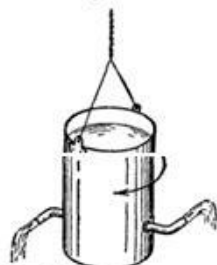
Рис. 320. Ведерко вращается в сторону, обратную направлению вытекания струи
