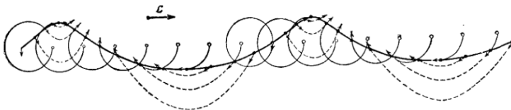
Рис. 437. Связь линий тока и круговых путей в бегущих водяных волнах. Горизонтальный ряд точек показывает частицы поверхности воды в состоянии покоя, дуги окружностей — пути, пробегаемые ими по направлению часовой стрелки. Соединив маленькие острия стрелок , мы получаем профиль распространяющейся вправо волны в конце следующего промежутка времени. Круговые траектории вычерчены для каждой второй стрелки.
