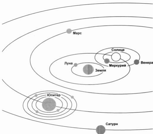
Система Тихо Браге
