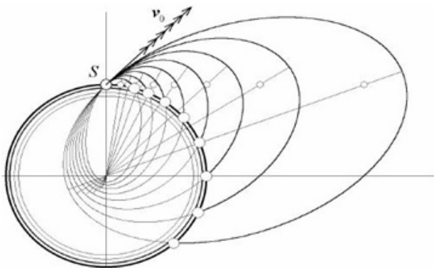
Семейство баллистических траекторий снарядов, запущенных с поверхности Земли под углом 45^\circ различными по модулю скоростями
